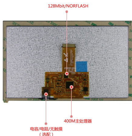
图 1-4 硬件配置图
