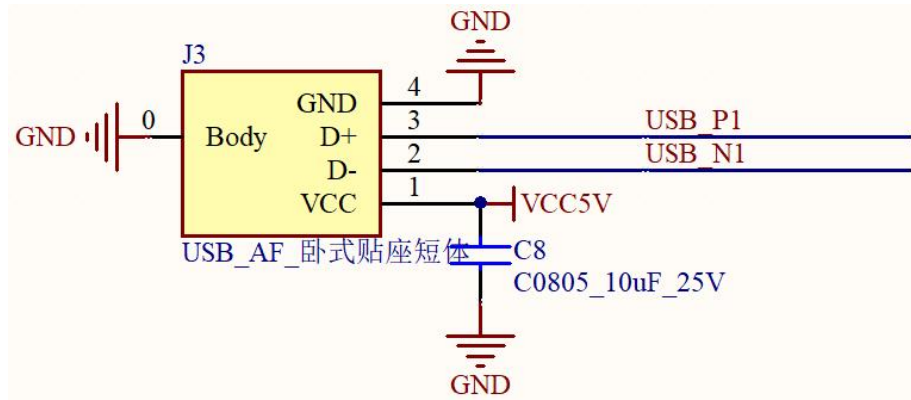
图 6-5U 盘参考电路
